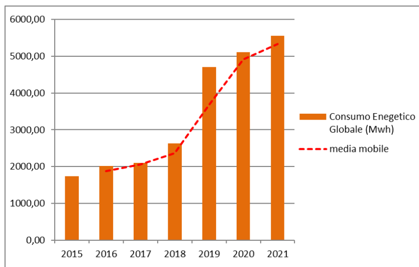
Figura 32 – Andamento sul consumo energetico globale dell'impianto, anni 2015-2021
