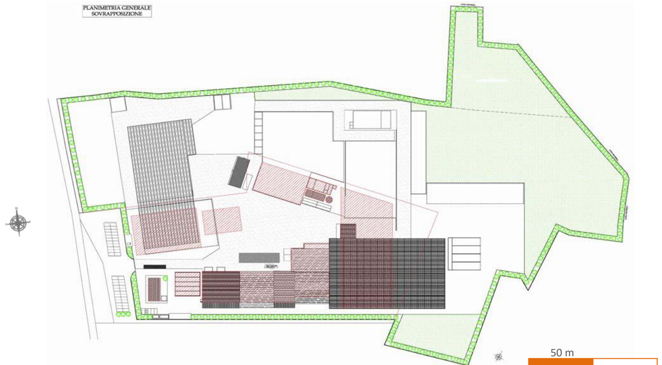
Figura 43 - Planimetria generale –sovrapposizione ante e post operam
