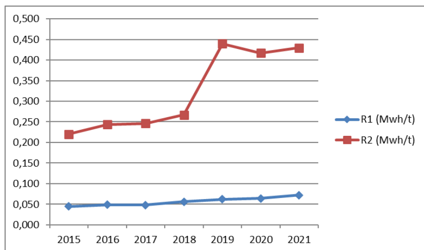
Figura 33 – Andamento indicatore sul consumo di energia elettrica, rapportato ai rifiuti in ingresso e al compost prodotto, anni 2015-2021
