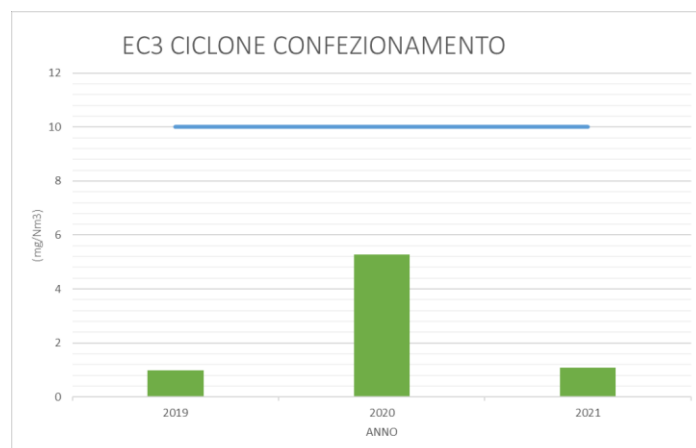
Figura 38 – Andamento sugli inquinanti emessi dal ciclone EC3, anno 2019-2021
