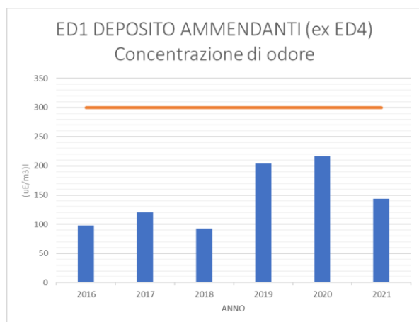
Figura 39 – ED1 valori di concentrazione di odore e polveri, rilevati in autocontrollo, anni 2016 - 2021
