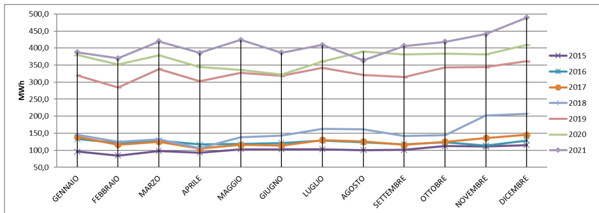
Figura 27 - Consumi elettrici mensili, nel periodo 2015-2021
