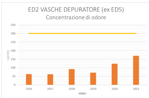
Figura 40 – ED2 valori di concentrazione di odore e polveri, rilevati in autocontrollo, anni 2016-2021
