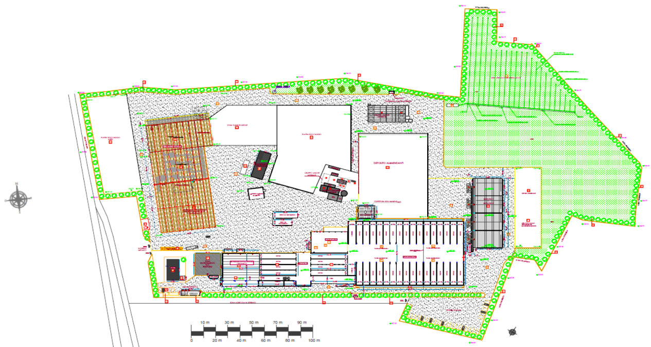
Figura 44 - Planimetria generale Primo stralcio funzionale al 31.12.2018
