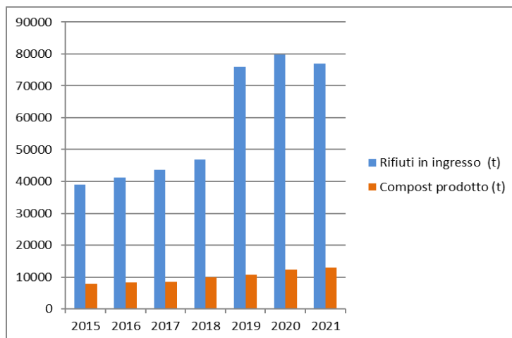
Figura 7 - Rapporto tra compost prodotto e rifiuti lavorati, nel periodo 2015-2021
