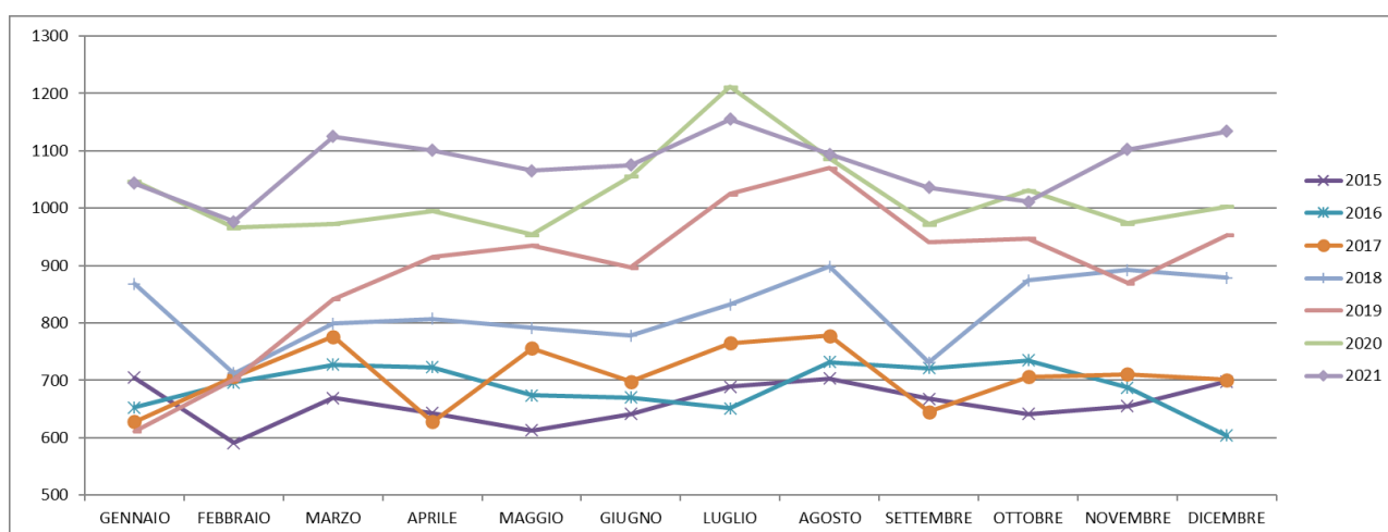
Figura 5 - Andamento su base mensile della produzione di compost (t/mese), nel periodo 2015-2021
