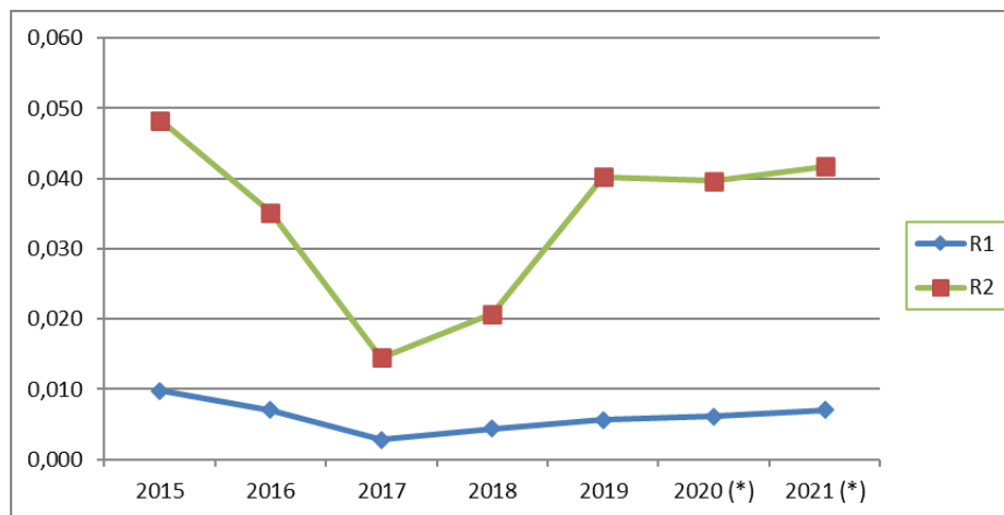
Figura 31 – Andamento indicatore sul consumo di e. e. rinnovabile, rapportato ai rifiuti in ingresso e al compost prodotto, anni 2015-2021
