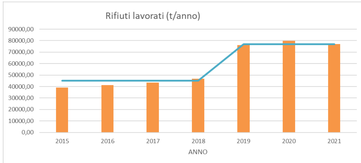
Figura 2 - Andamento annuo dei quantitativi di rifiuti lavorati, nel periodo 2015-2021
