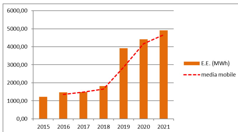
Figura 28 – Andamento sul consumo di energia elettrica, anni 2015-2021
