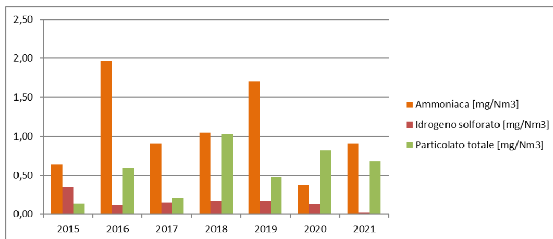
Figura 36 – Andamento sugli inquinanti emessi dal biofiltro EC1, anni 2015-2021
