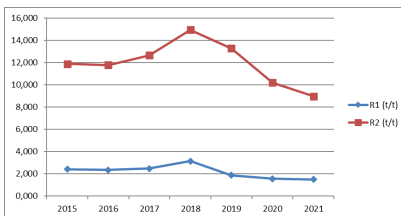
Figura 26 – Andamento indicatore sul consumo di gasolio rapportato ai rifiuti in ingresso e al compost prodotto, anni 2015-2021
