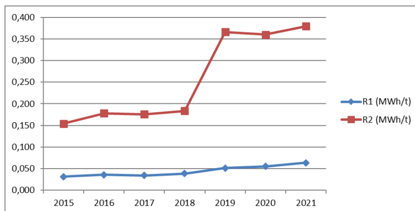
Figura 29 – Andamento indicatore sul consumo di energia elettrica, rapportato ai rifiuti in ingresso e al compost prodotto, anni 2015-2021
