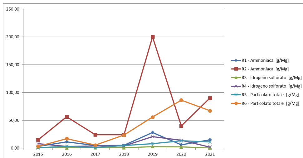
Figura 37 – Andamento indicatori sugli inquinanti emessi dal biofiltro EC1, rapportato ai rifiuti in ingresso e al compost prodotto, anni 2015-2021
