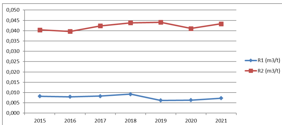
Figura 22 – Rapporto indicatori consumi idrici/rifiuti in ingresso [R1] e consumi idrici/compost prodotto [R2], anni 2015-2021
