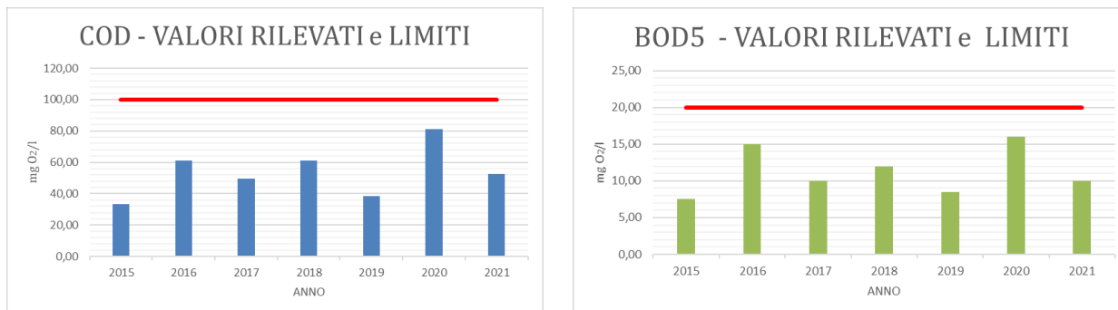
Figura 23 – Confronto valori COD e BOD5 rilevati in autocontrollo con limiti di legge, anni 2015-2021
